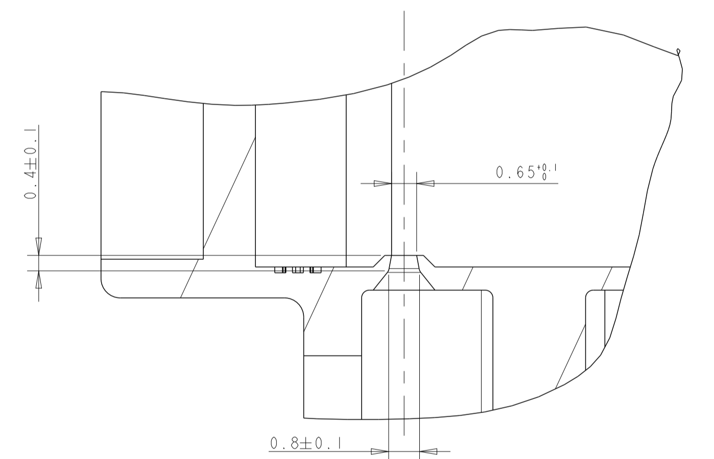
COUPE C-C DETAIL ALVEOLE MPQ ECHELLE 10:1
