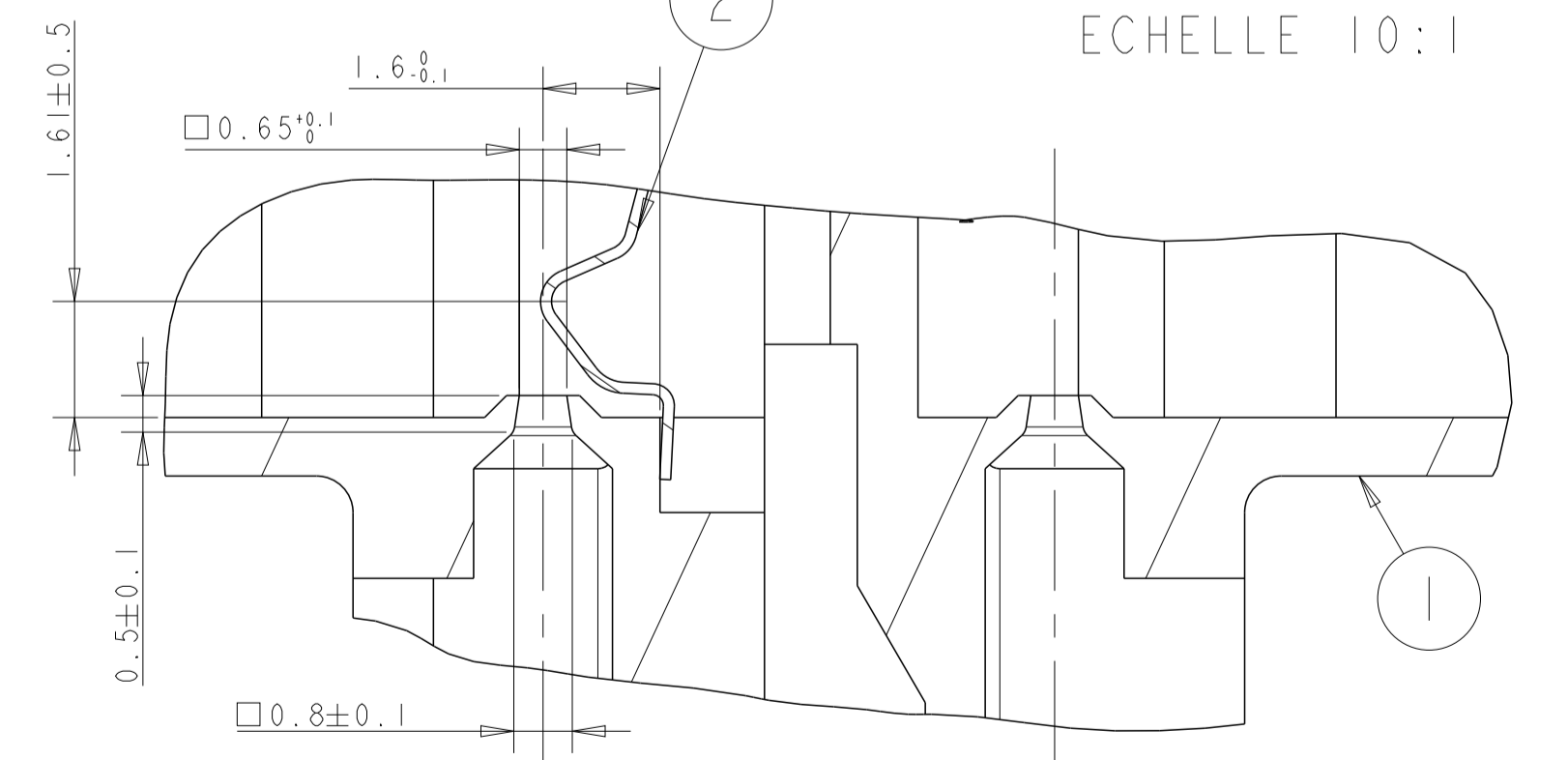
COUPE D-D DETAIL ALVEOLE MQS ECHELLE 10:1
