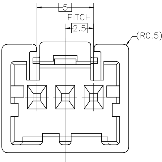
SECT A-A
