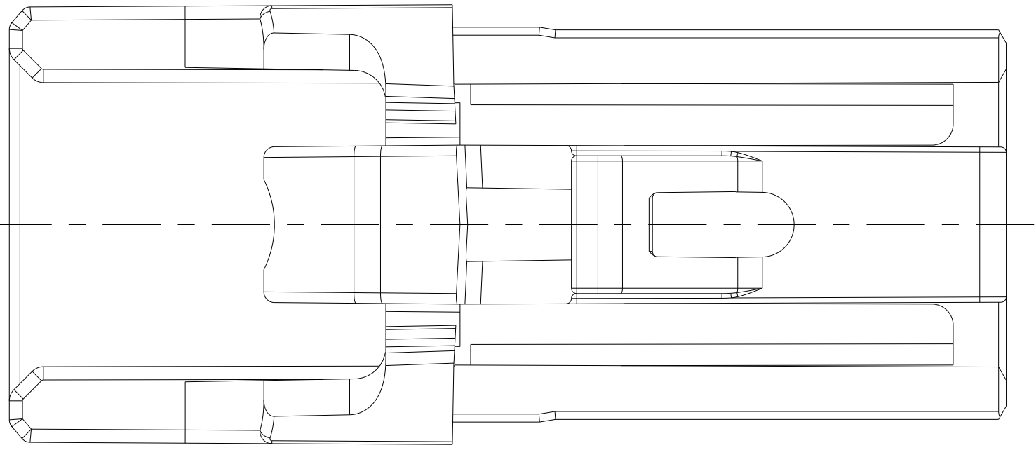
CODINGS, PLUG SIDE, SIMILARITY AS VIEW SCALE 5:1 Kodierung, Steckseite, Darstellung der Kodierungen nur aehnlich
