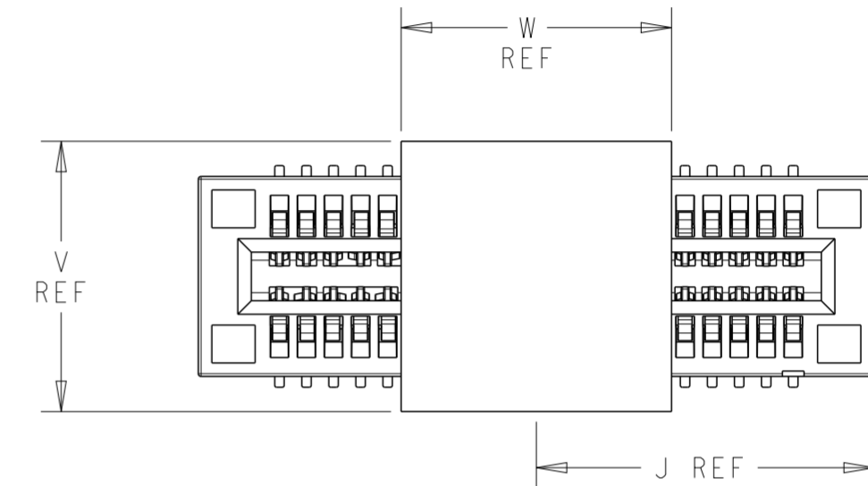
MYLAR SIZE SCALE 4:1
