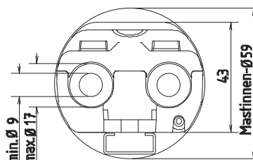
Kabelzugang
