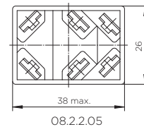
2- POLE (depth 41.5)
