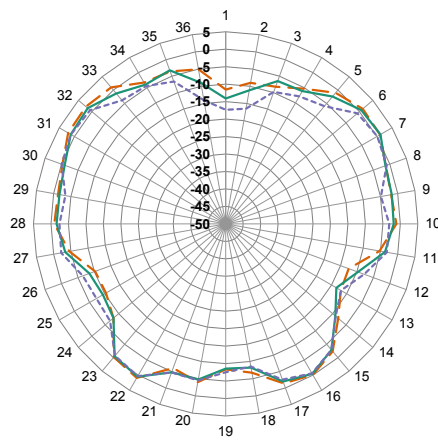
YZ-Plane Gain
