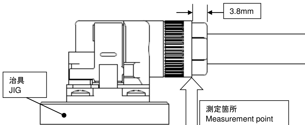
Fig.6 コネクタ保持力 Fig.6 Connector retention force
