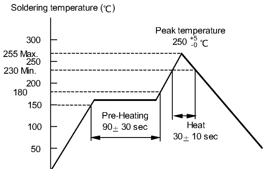
Fig.2 リフロー半田の温度プロファイル Fig.2 Temperature Profile of Reflow Soldering
