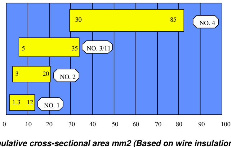
ES2000 TUBING SIZE RANGE TABLE
