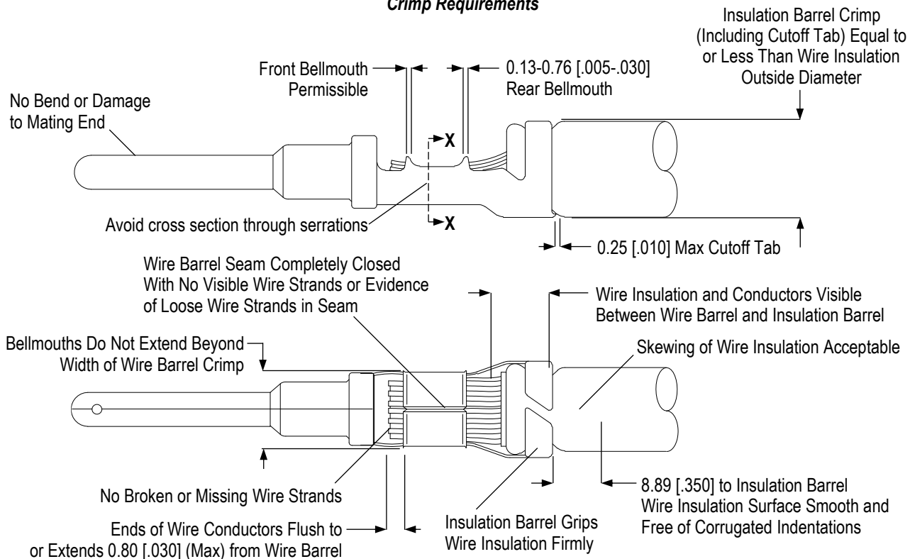
Wire Size 14 AWG SXL (SAE J1128) Shown
