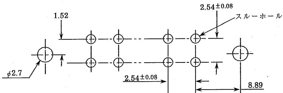
Fig. 2 スルーホールレイアウト
