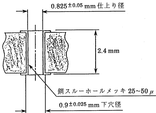
Fig. 3 スルーホール径
