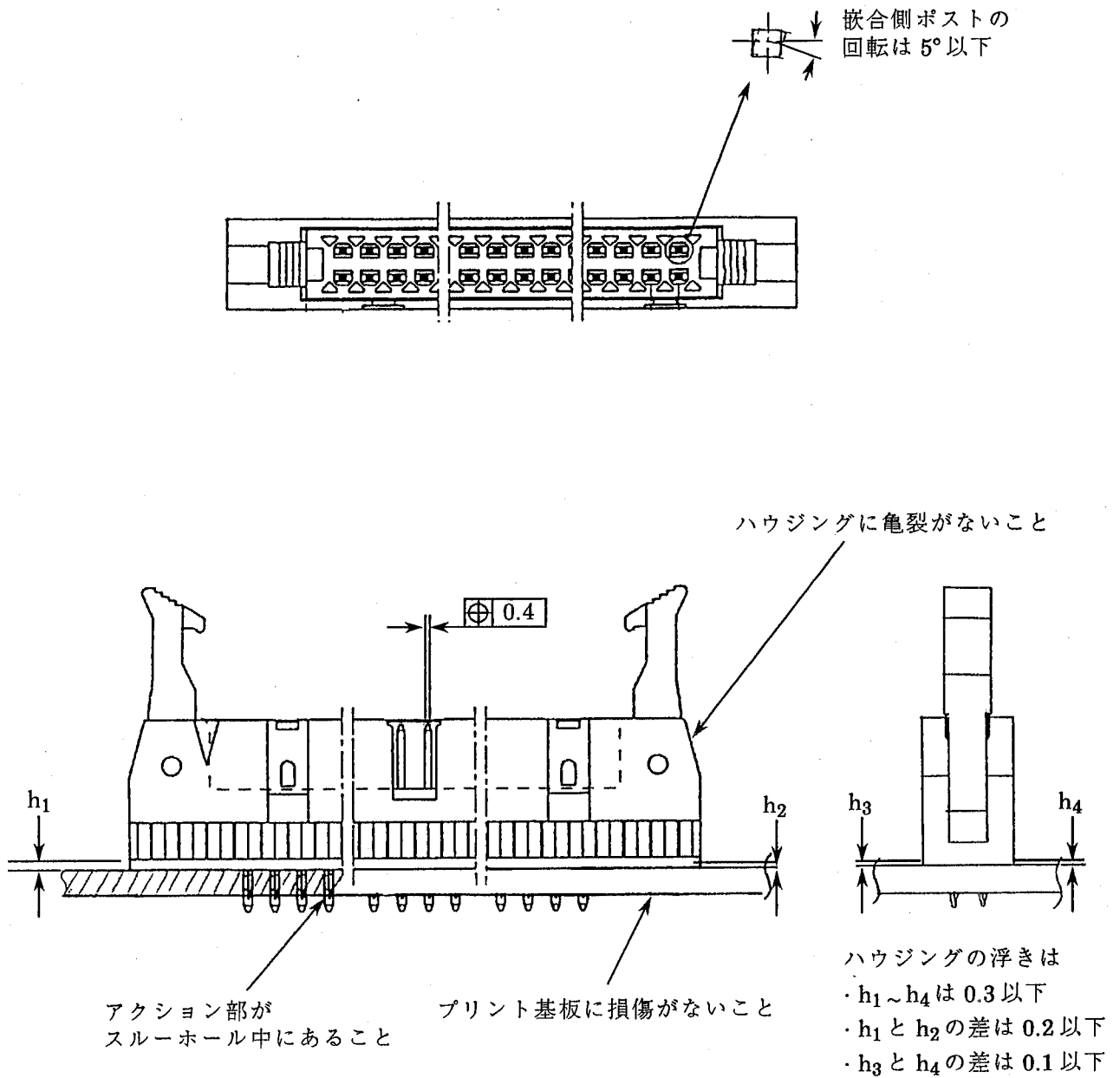
Fig. 4 圧入後の必要条件
