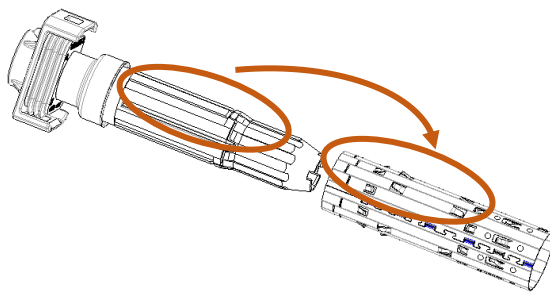
Figure 9: Assembly sequence/Montagereihenfolge
