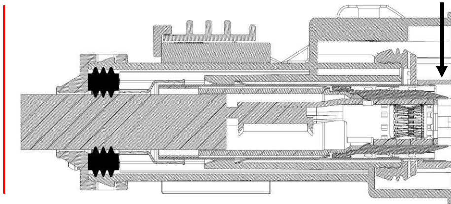
Figure 20: Cross section through locking latch Querschnittsdarstellung durch die 2.Kontaktsicherung
