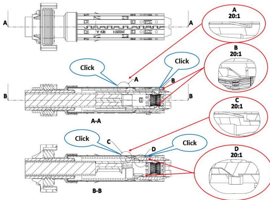
Figure 10: Plugged positions/Verrastungspositionen/
