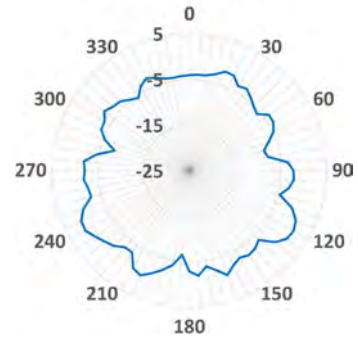
YZ-5.3GHz
