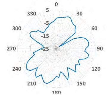
XZ-5.8GHz
