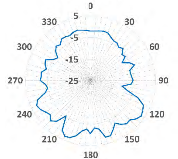
YZ-5.8GHz
