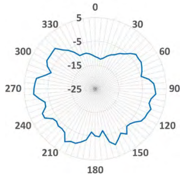
YZ-5.2GHz
