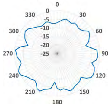
YZ-5.2GHz
