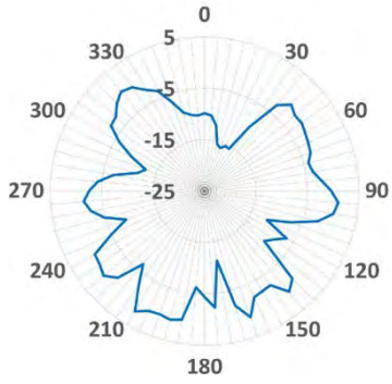
XZ-5.2GHz
