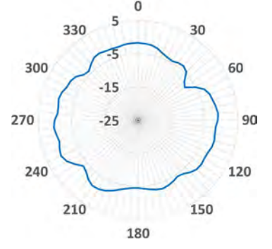
XY-5.2GHz
