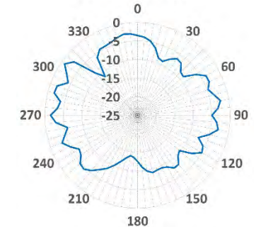
XY-5.8GHz
