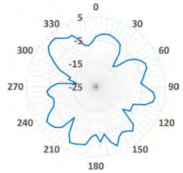
XZ-5.3GHz
