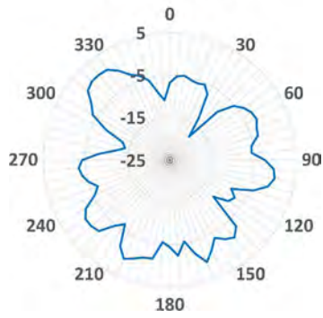
XZ-5.2GHz
