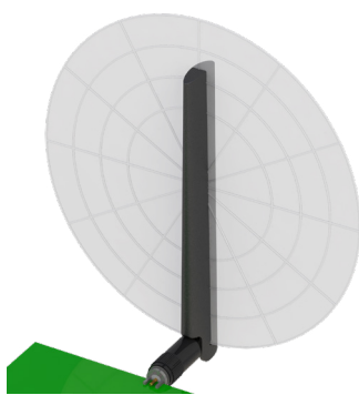
XZ-Plane Gain
