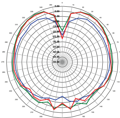
YZ-Plane Gain
