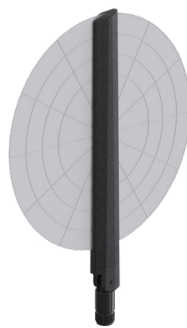
YZ-Plane Gain
