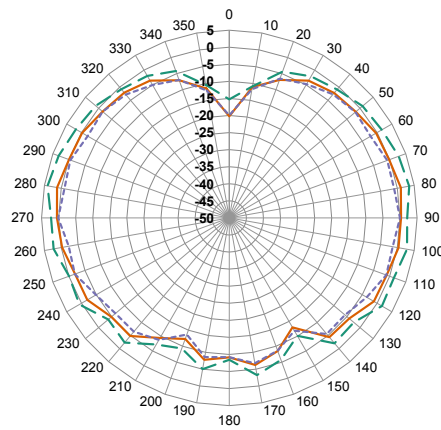
YZ-Plane Gain
