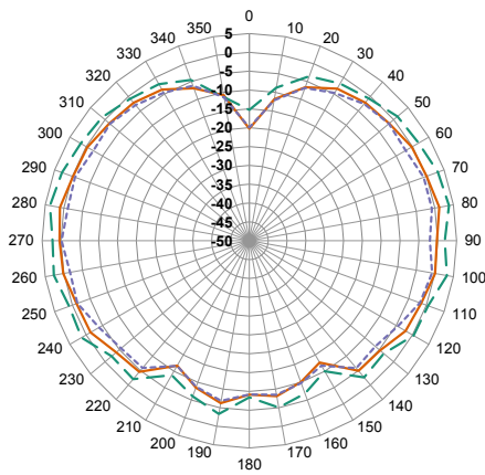
XZ-Plane Gain
