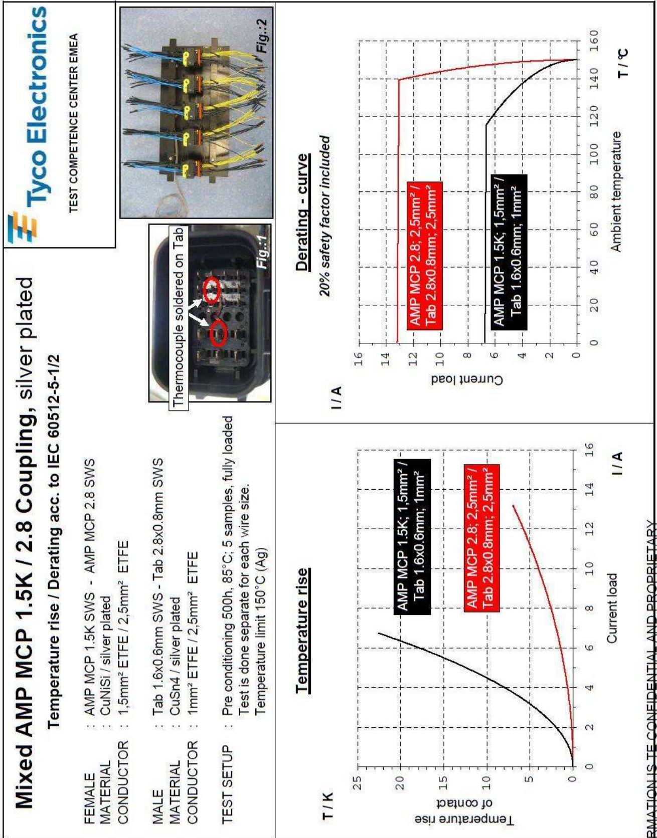
Fig. / Abb. 3.5.1: Coupling, 22pos., silver-plated contacts / 22polige Kupplung mit versilberten Kontakten
