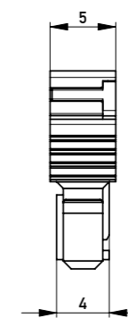
Abdeckung verpresst
