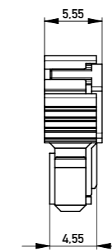
Abdeckung vorverrastet
