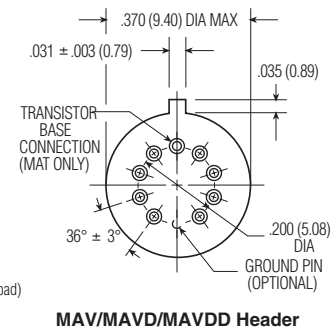
MAV/MAVD/MAVDD Header
