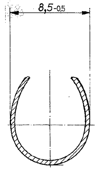
SCHNITT B-B
