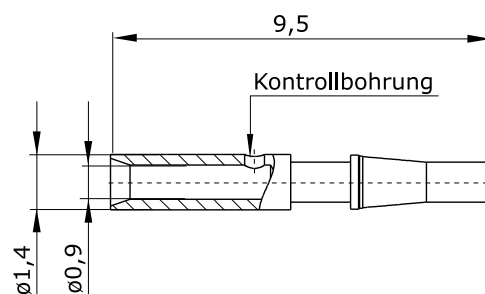
Hauptabmessungen Kontaktbuchse
